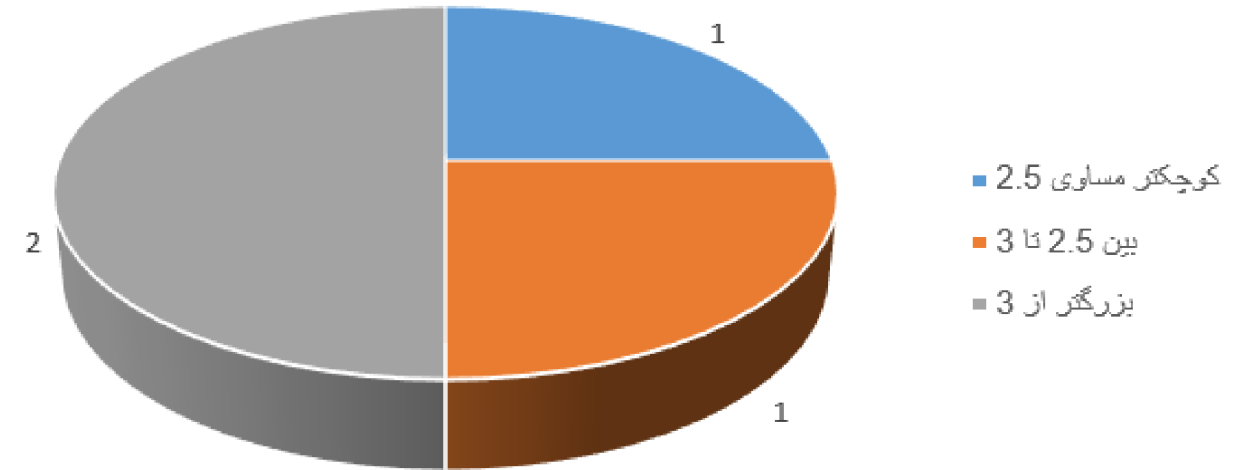
مشخصات زمین لرزه های خرداد ماه ۱۴۰۳
